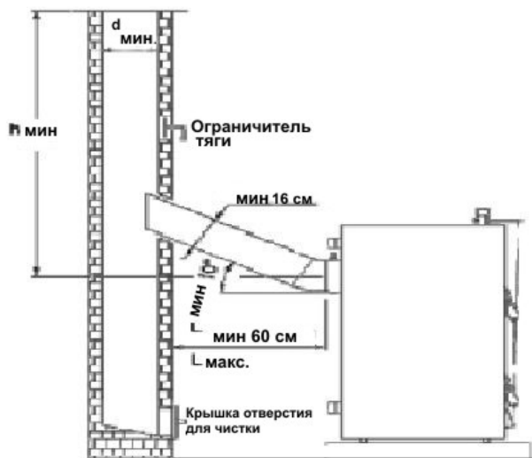
Рис. 6 Пример подключения к дымоходу
